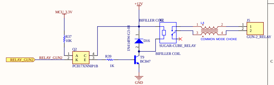
GUN-2_RELAY
